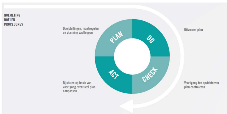
Fig. 1 PDCA-Cirkel Deming
